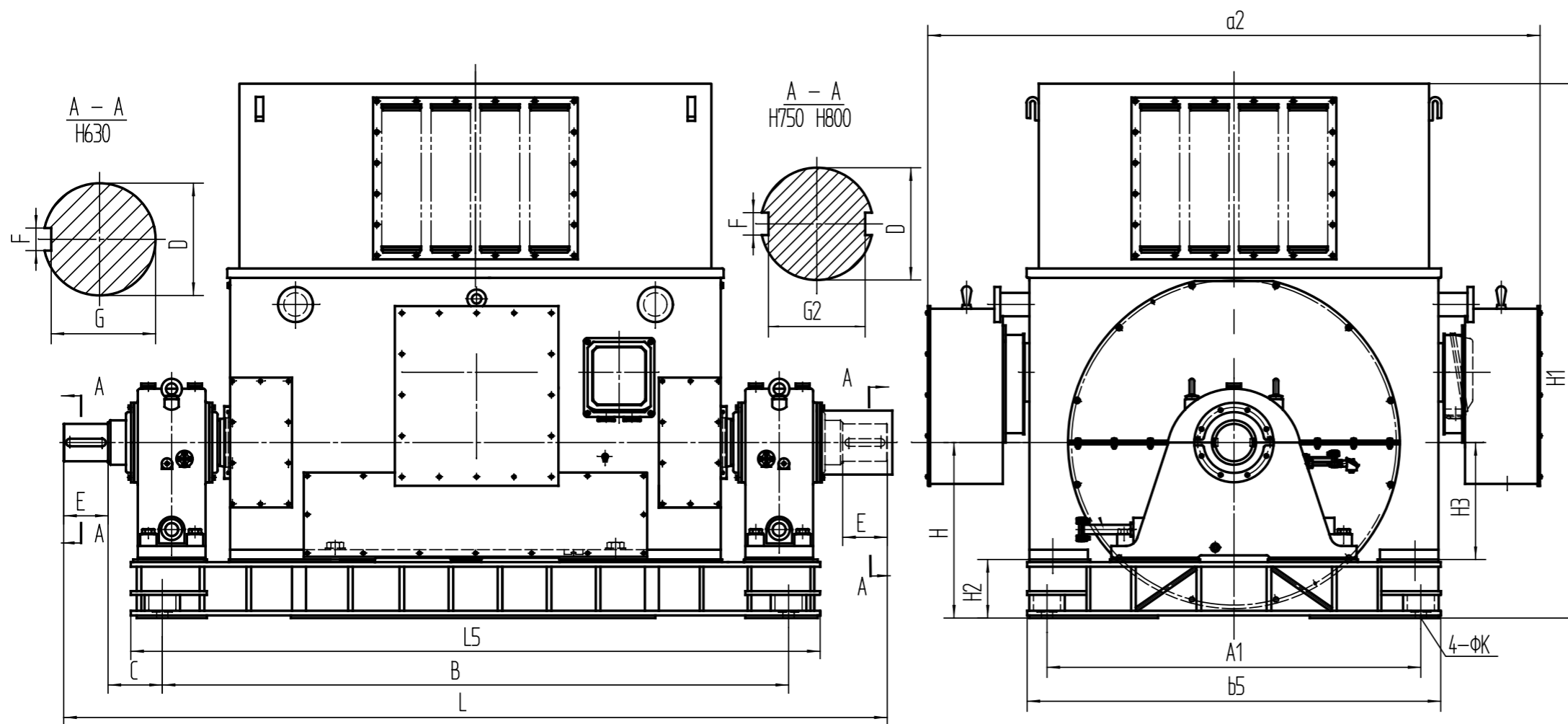
YK 系列安装尺寸表(6000V、10000V IP23)
